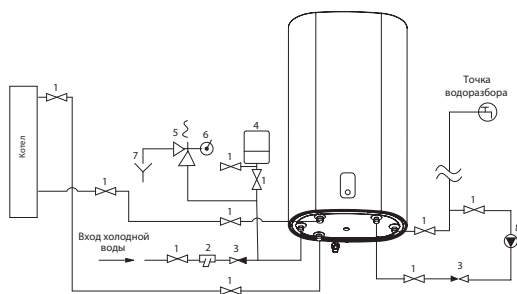
Рис. 4. Вертикальная схема
